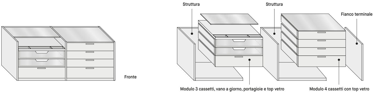
Esempio struttura affiancata/invertita
