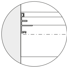
Sezione anta vetro
