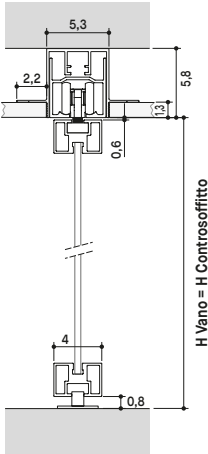
Struttura portante **
