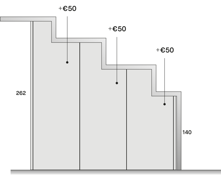
ESEMPIO TAGLIO A SCALA
