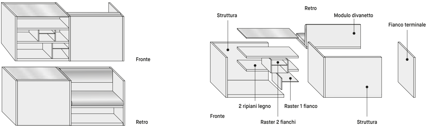
Esempio struttura affiancata/invertita
