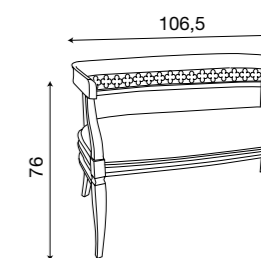
L. 106,5 P. 54 H. 76 seduta H. 46
